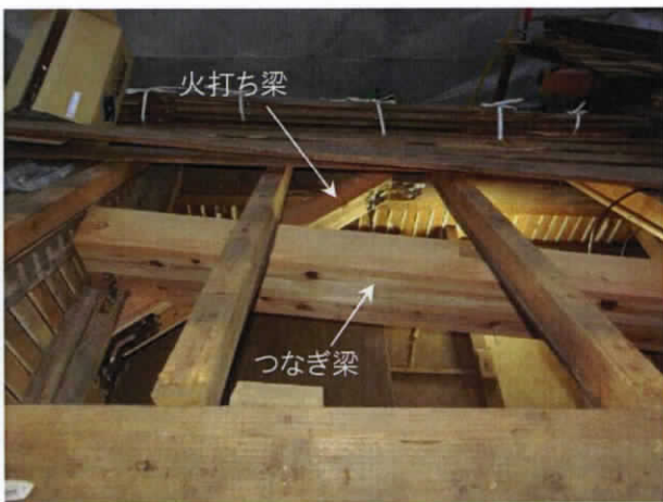
火打ちとつなぎ梁の取付状況
