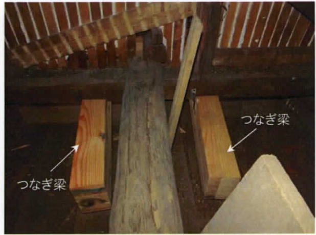
つなぎ梁取付状況(水屋側)
